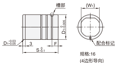
导套
