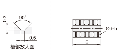
滚针衬套
