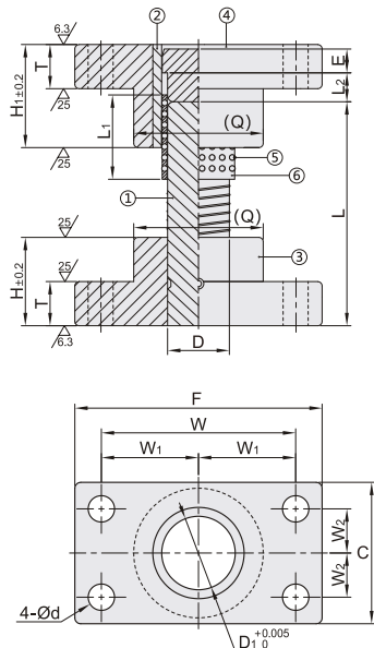
无定位孔型 AOFH45/46/73/74
