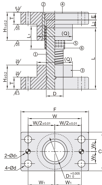
定位孔型 AOFH35/36/47/48
