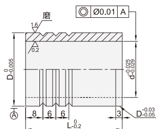
厚壁直柱型 AOFF51
