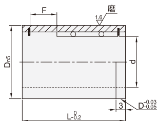
压入型·直柱型 AOFF01
