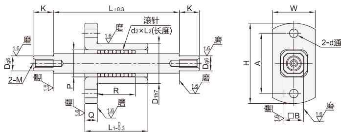
两端内螺纹型 ALOK02
