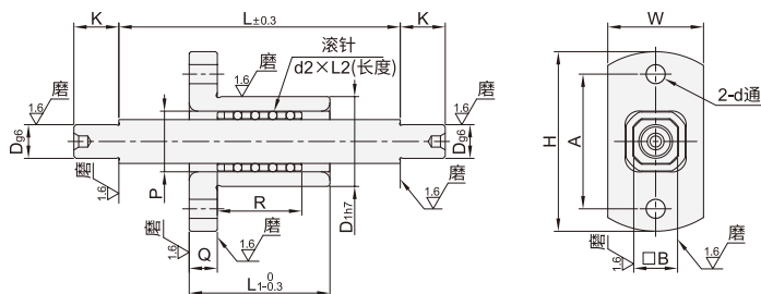
无螺纹型 ALOK01
