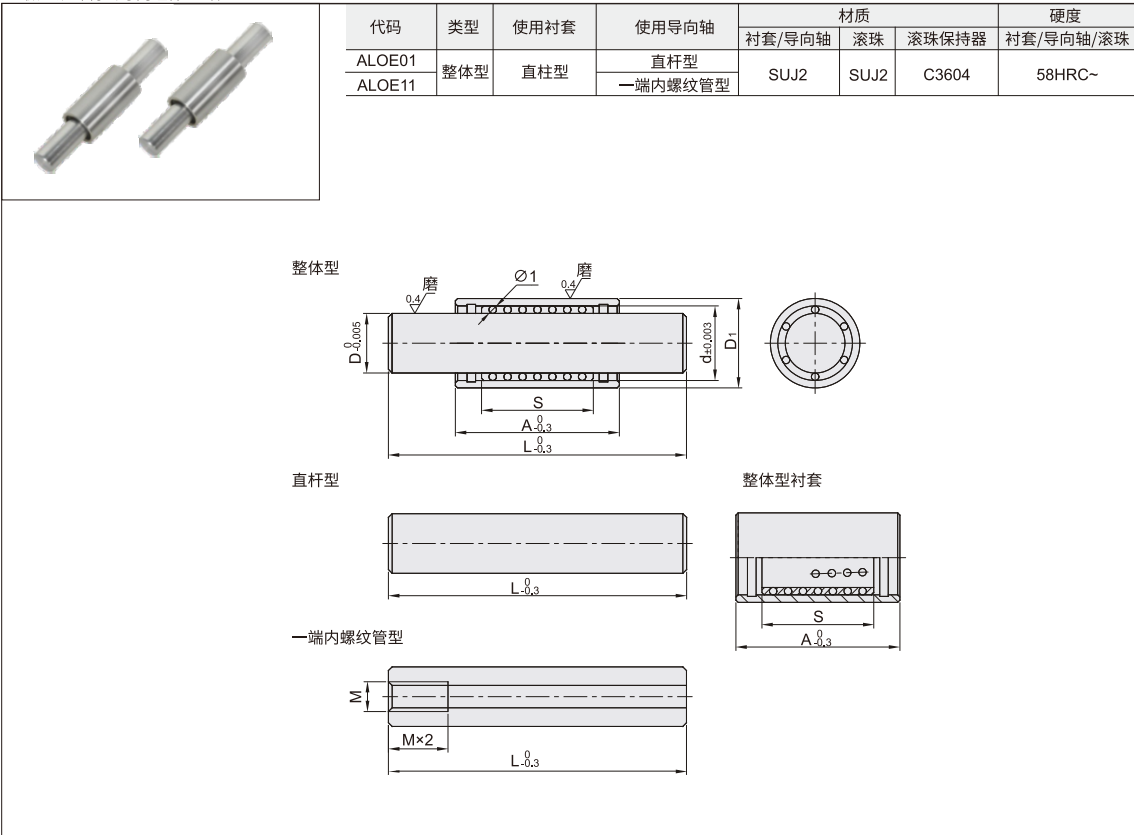
■微型滚珠衬套导向组件·整体型
