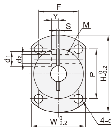
对边法兰型ZPM11/12/16
