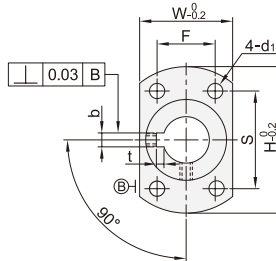
对边法兰型 ZPU11/12
