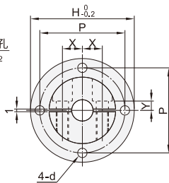
圆法兰型 ZPY01/02/06
