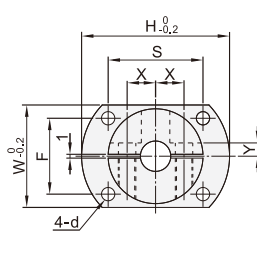
对边法兰型 ZPY11/12/16
