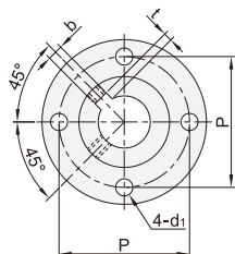
圆法兰型 ZPY01/02/06
