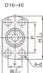
对边法兰型 ZPF21/22/26
