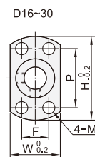
对边法兰型 ZPC21/22/26
