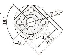
方法兰型 ZPC11/12/16
