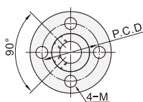
圆法兰型 ZPC01/02/06
