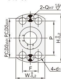
对边法兰型 ZPU31/32/33
