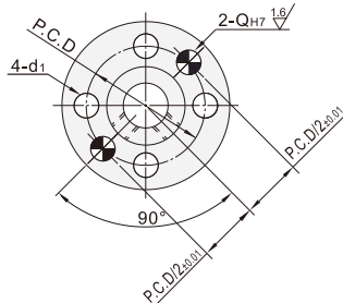
圆法兰型 ZPU01/02/03
