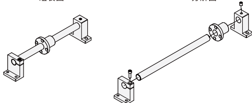
组装图
