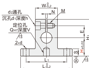
带定位孔 ZTU03
