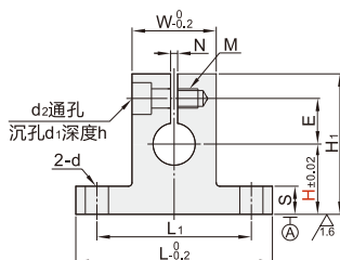
无定位孔 ZTU01/02
