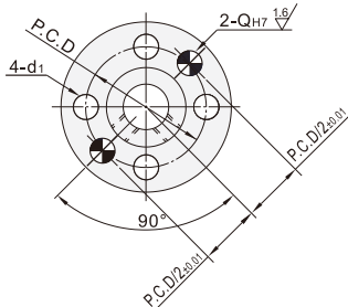
圆法兰型 ZPU01/02/06
