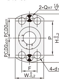
对边法兰型 ZPU31/32/36
