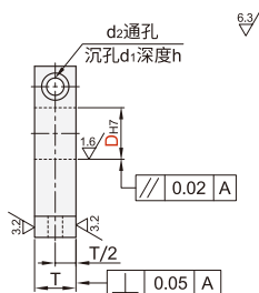
轴环部详图
