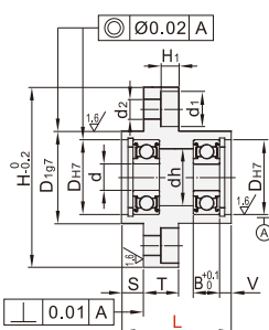
圆法兰
