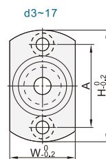
对边法兰
