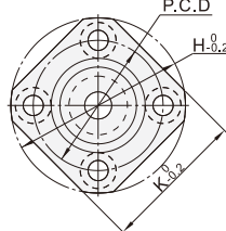
方法兰
