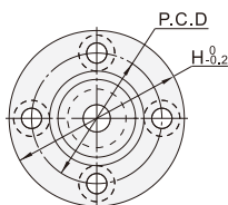
圆法兰
