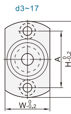
对边法兰
