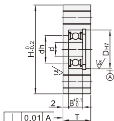
带扣环型
