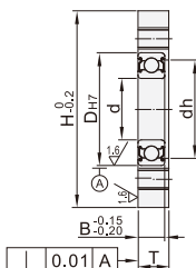
无扣环型
