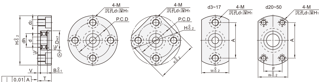
圆法兰 BTE01/02/03/04/05
