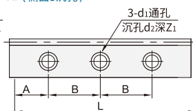
HP(侧面3沉孔)
