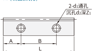
HF(侧面2沉孔)
