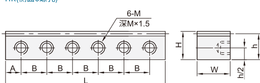
HR(侧面6螺孔)
