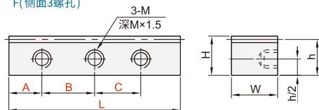
F(侧面3螺孔)
