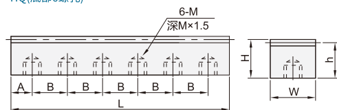
HR(侧面6螺孔)
