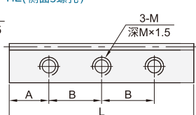
HE(侧面3螺孔)
