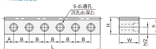
HS(侧面6沉孔)
