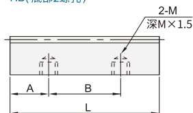
HD(侧面2螺孔)
