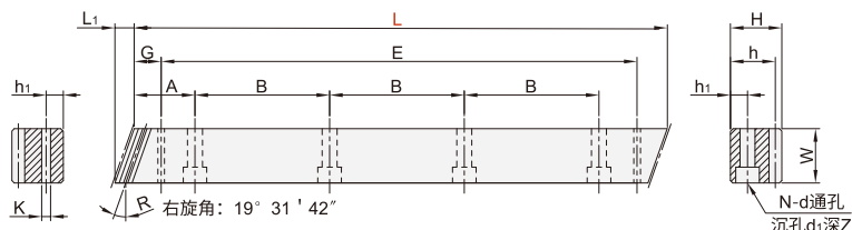
■端面尺寸图
