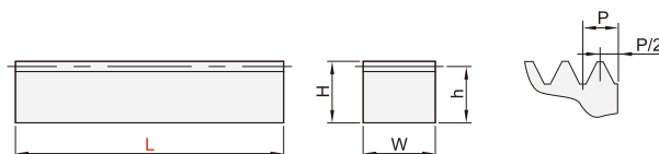
■端面尺寸图
