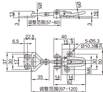
安装孔孔距
