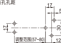
安装孔孔距
