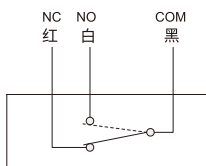
接线图
