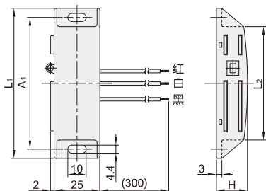
四磁芯 VPH67
