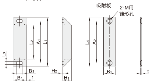
长条防尘型 VPG66
