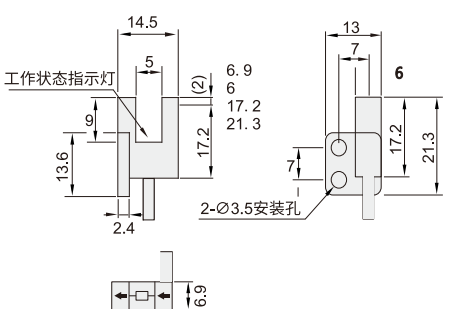
RU2-FN45 RU2-FP45
