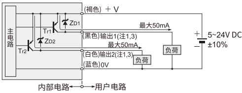
输出: RU2-P45
