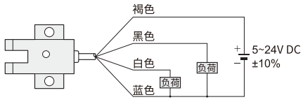
线路图
