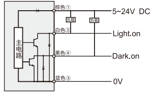
输出: RU2-N45
