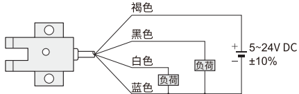
线路图
