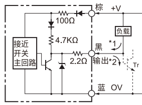
PNP输出
