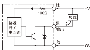
NPN输出
