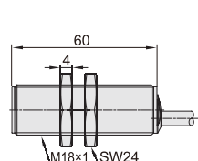
导线式M18
