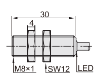
导线式M8
