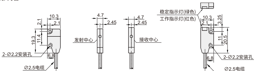
侧面出光尺寸图
