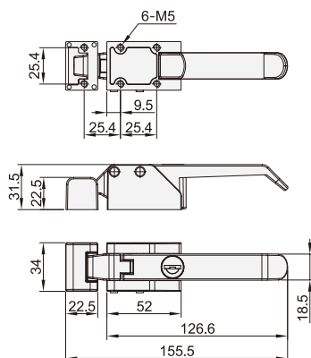
把手型 FAS11/12
