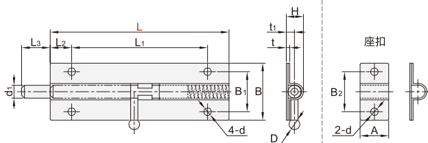
带弹簧装置,标准型 FAY11
