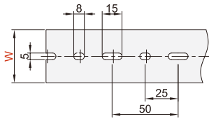
W≤60mm线槽底部孔尺寸
