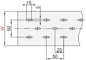
W≥80mm线槽底部孔尺寸
