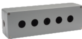
五孔铝盒 188×120×80mm JAXG14-05G
