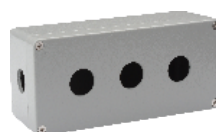
三孔铝盒 175×80×56mm JAXG14-03
