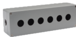
六孔铝盒 188×120×80mm JAXG14-06G
