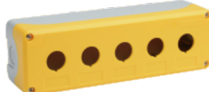
五孔 230×70×60mm JAXG12-5-Y
