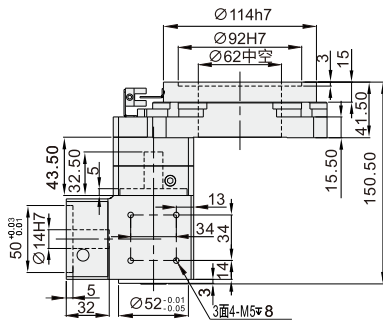
K向视图
