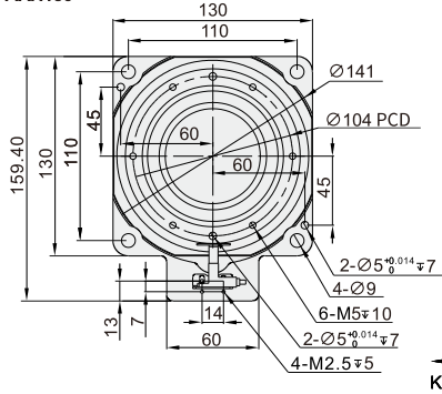
K向
