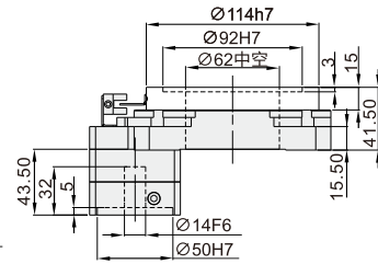
K向视图
