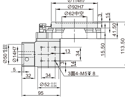
K向视图
