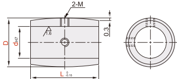
圆弧型 LBF33/LBF34
