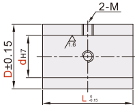
带止动螺丝型 直柱形 LBF03/LBF04
