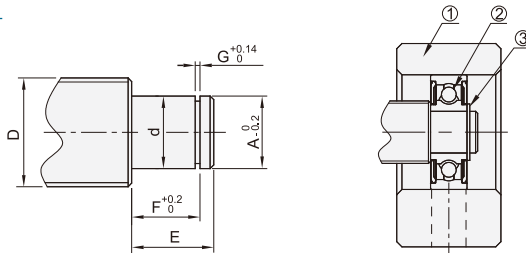
参考轴端加工尺寸
