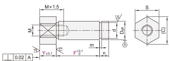
六角型 MXC21/22/26
