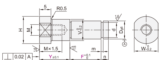
台阶型 MXC11/12/16
