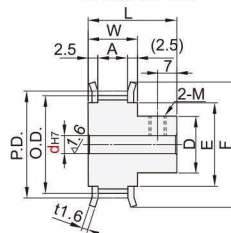
带轮形状: B形
