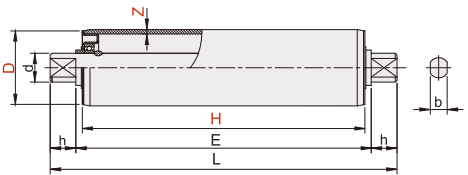
对位铣扁型 LDP21 LDP22 LDP23
