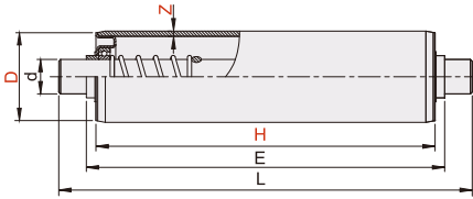
弹簧嵌入型 LDP01 LDP02 LDP03
