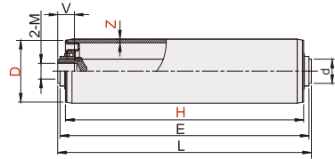
内螺纹型 LDP11 LDP12 LDP13
