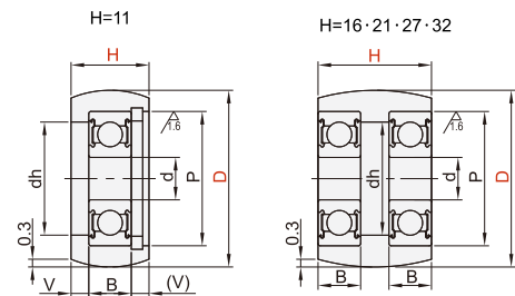
圆弧型 VBG21/22/24/31/36
