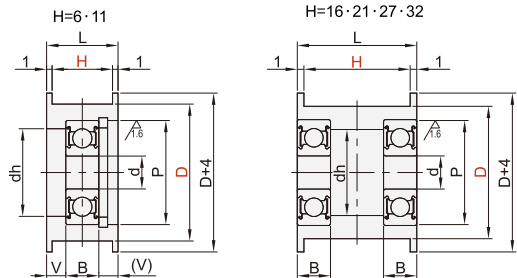
法兰型 VBG01/02/04/11
