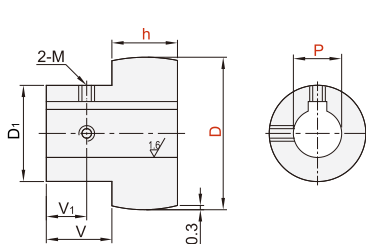
圆弧形 VBC11/12/13/14
