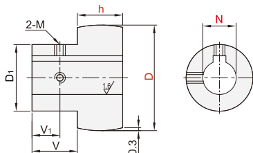
圆弧型 VBC11/12/13/14
