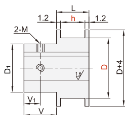
法兰型 VBC01/02/03/04
