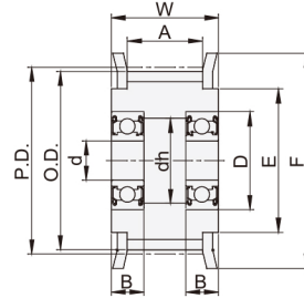
VTH01 双轴承
