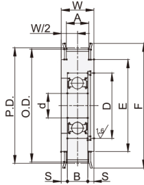
VTP01 单轴承
