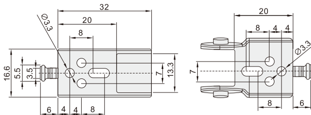
B款 外开10×10
