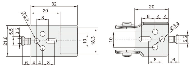
外开10×15
