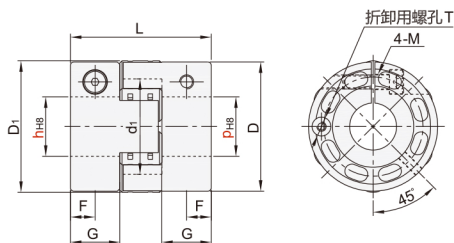
CEC21 CEG21 螺钉夹紧型
