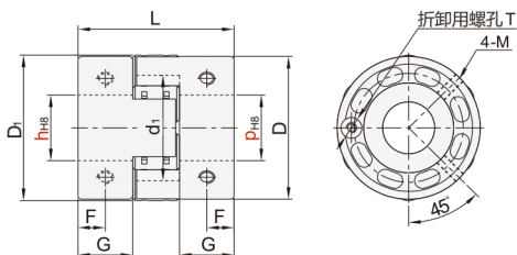
CEC01 CEG01 螺钉固定型
