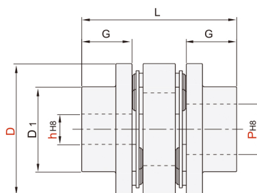
CDP21 CDQ21 双膜片
