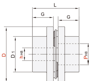
CDP01 CDQ01 单膜片
