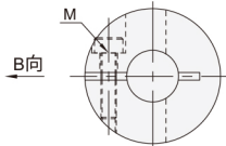
B向视图
